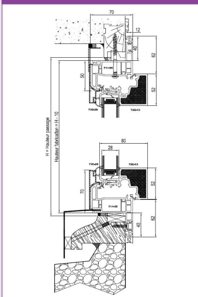
Ailette rénovation de 40 mm de série
