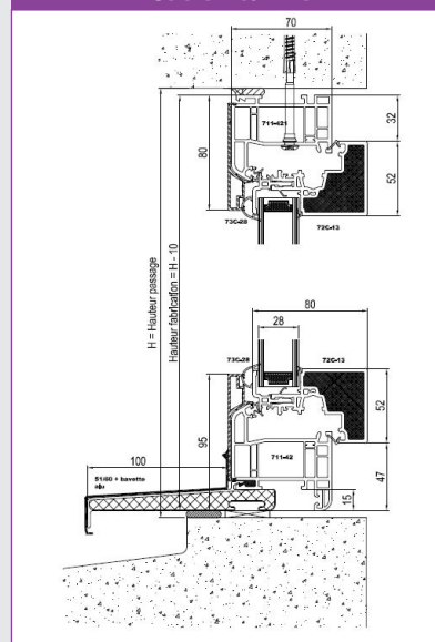
Dormant de 70 mm et pièce d'appui rapportée dépassant de 100 mm de série
