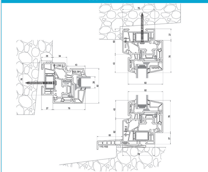
Dormant de 76 mm et pièce d'appui rapportée de 60 mm
