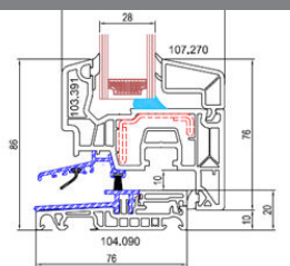
Seuil aluminium à rupture de pont thermique avec gâche encastrée
