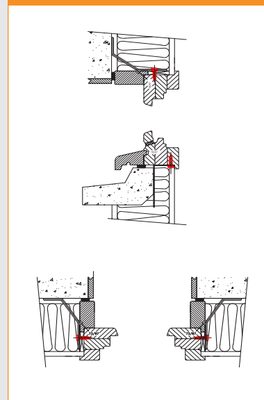
Isolation intérieure de 65 mm sans tapée Isolation intérieure de 100-120-140-160 avec tapées (option appui débordant)
