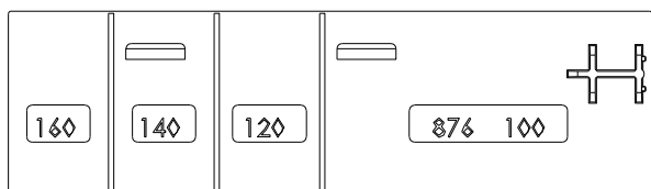
Embouts dormant 76100L-76120L-76140L-76160L H&amp;B 8761X0 (PA)
