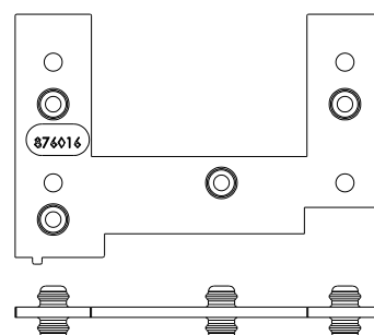
Embout dormant 76120HVR-76140HVR 876016
