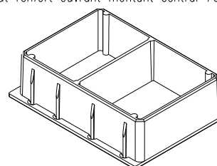
Embout renfort ouvrant montant central 76312 876312 (PA)
