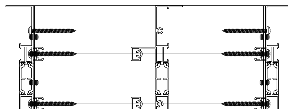
Assemblage traverse haute par vis VAT-S-7049-SR2-4.8x50
