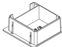
Embout renfort ouvrant montant central 76306 876306 (PA)
